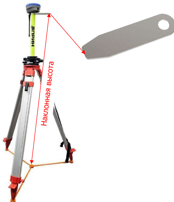
Рис. 1.4 Наклонная высота
