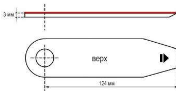
Рис. 1.5 Выносная пластина для измерения наклонной высоты антенны
